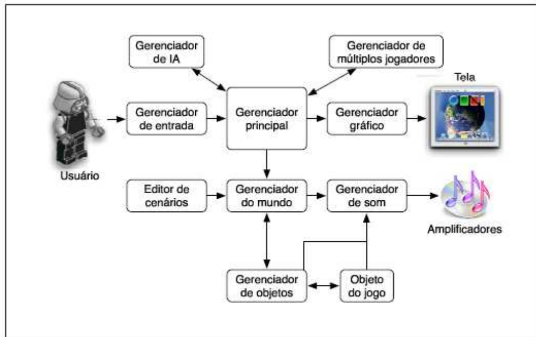
Figura 14 – Arquitetura genérica de um jogo de computador
